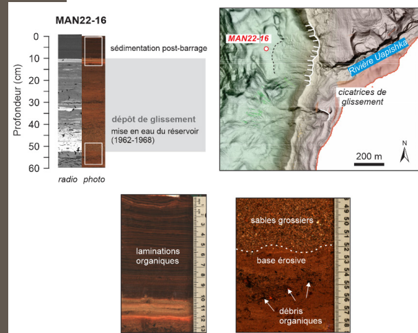
Figure 2. Cicatrices de glissements à l'embouchure de la rivière Uapishka (voir localisation sur la Figure 1) [1]. Les dépôts associés forment une épaisse couche de sédiment à base sableuse érosive dans la carotte MAN22-16, avec notamment des niveaux denses (blancs) sur l'image radiographique. Cet événement précède le début de la sédimentation laminée organique associée au réservoir [3].
