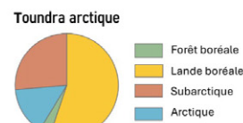
Figure 1. Répartition des groupes phytogéographiques de la flore de la tundra arctique et des landes sommitales de quatre secteurs de la zone boréale au Québec (Caniapiscou-nord, Caniapiscou-sud, Fermont, monts Uapishka).
