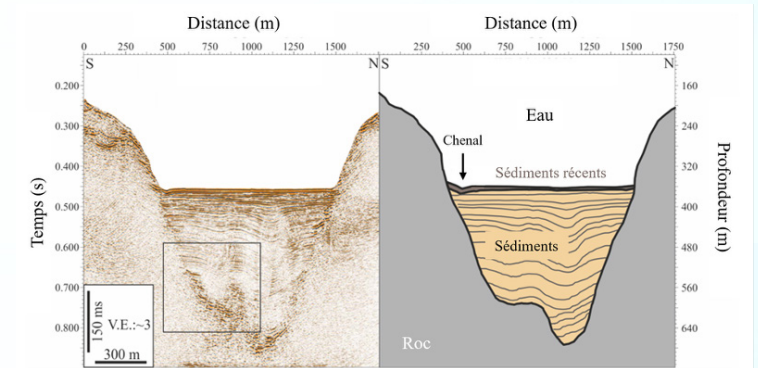
Figure 4. Profil sismique AWI2016-8250 (gauche) et schéma interprétatif (droite) de la vallée creusée dans le roc et du remplissage ultérieur par des sédiments (épaisseur maximale de 300 m) dans le secteur amont du lac (voir localisation sur Figure 1) [4].
