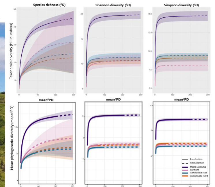
Figure 2. Courbes de raréfaction et extrapolation des nombres de Hill de la diversité taxonomique et des indices de la diversité phylogénétique moyenne de Faith dans les landes sommitales de quatre secteurs en forêt boréale au Québec (monts Uapishka, Fermont, Caniapiscou-sud, Caniapiscou-nord). Les ombrages indiquent les intervalles de confiance à 95%.
